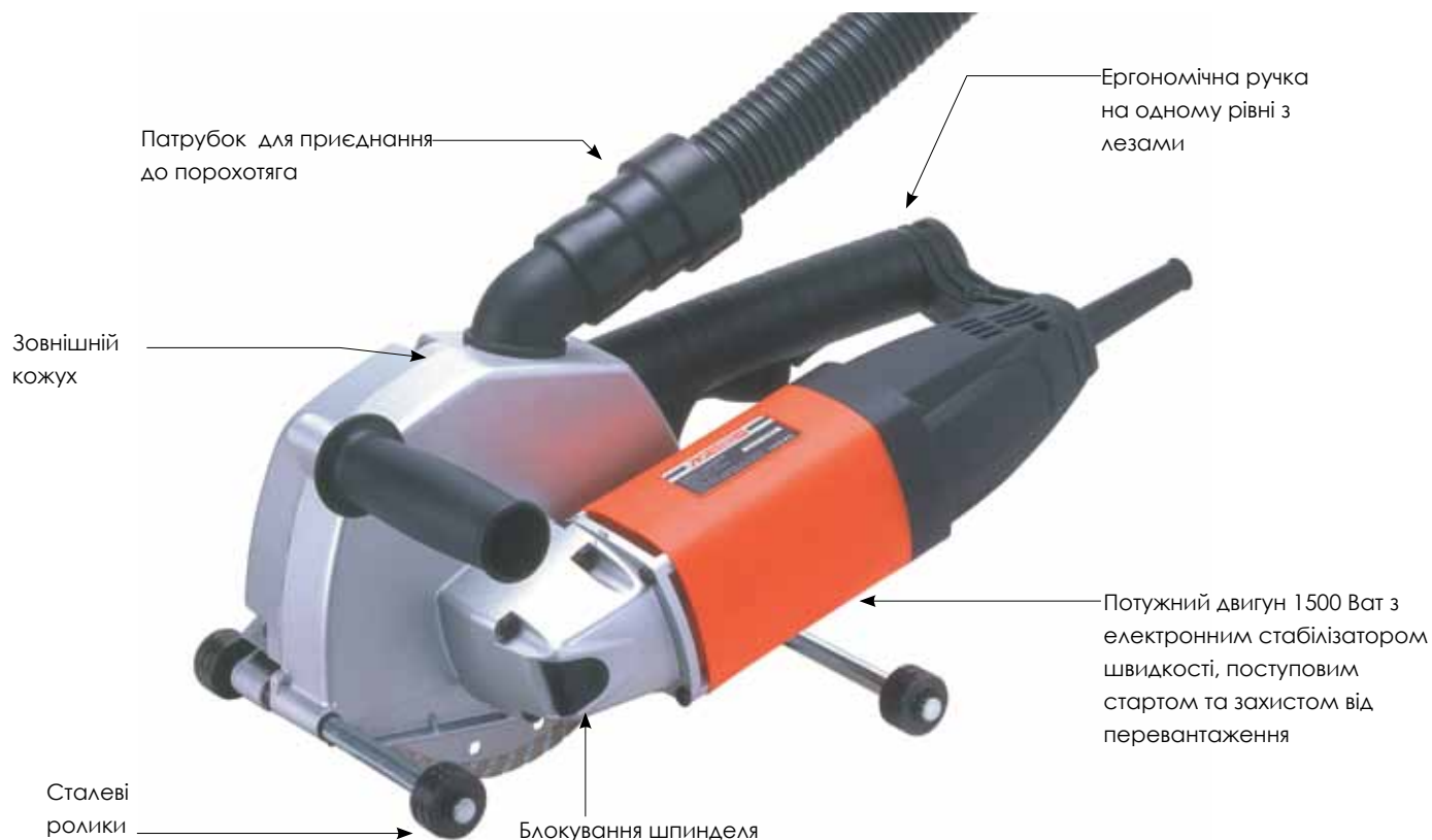
CS 150 (з регульовальними фланцями)
